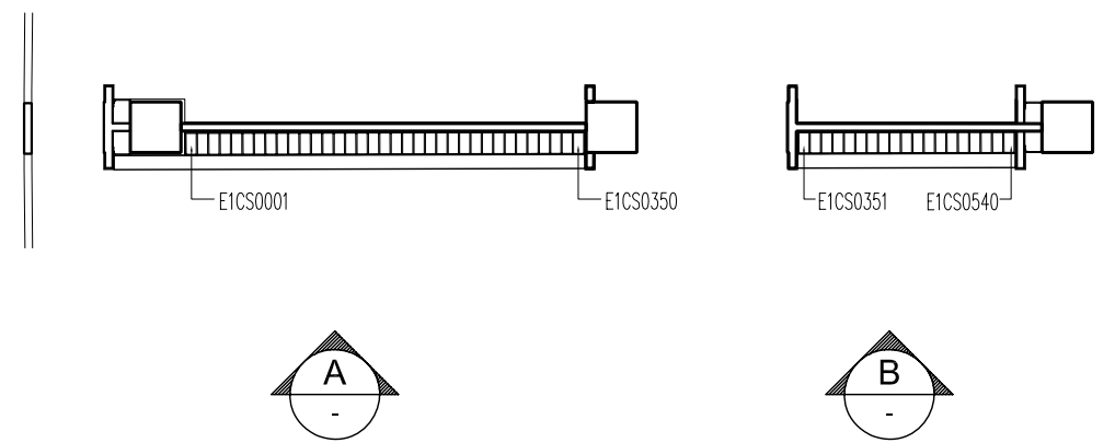
一樓平面圖
