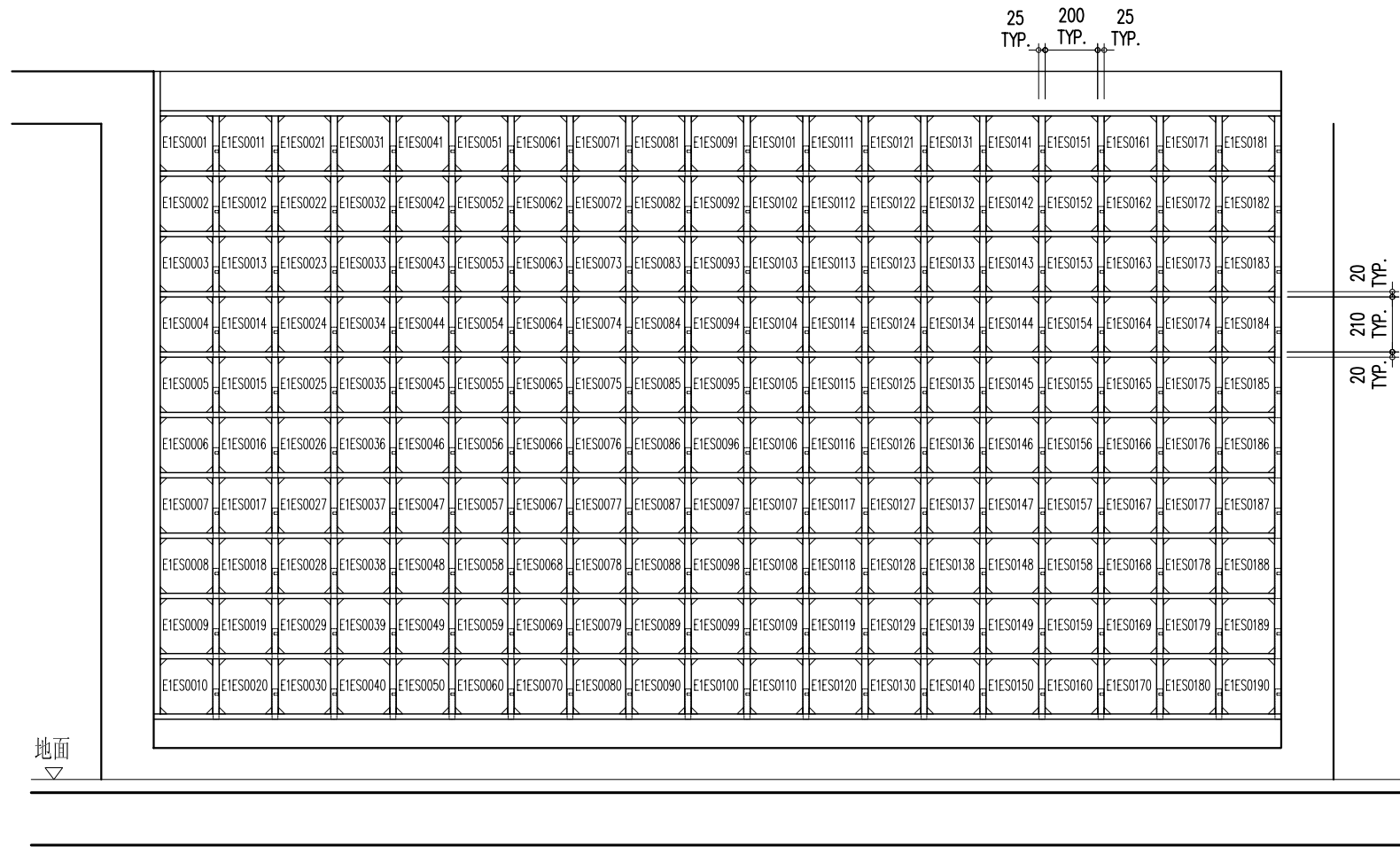
E1ES0001 ~ E1ES0190 一樓立面圖 A
