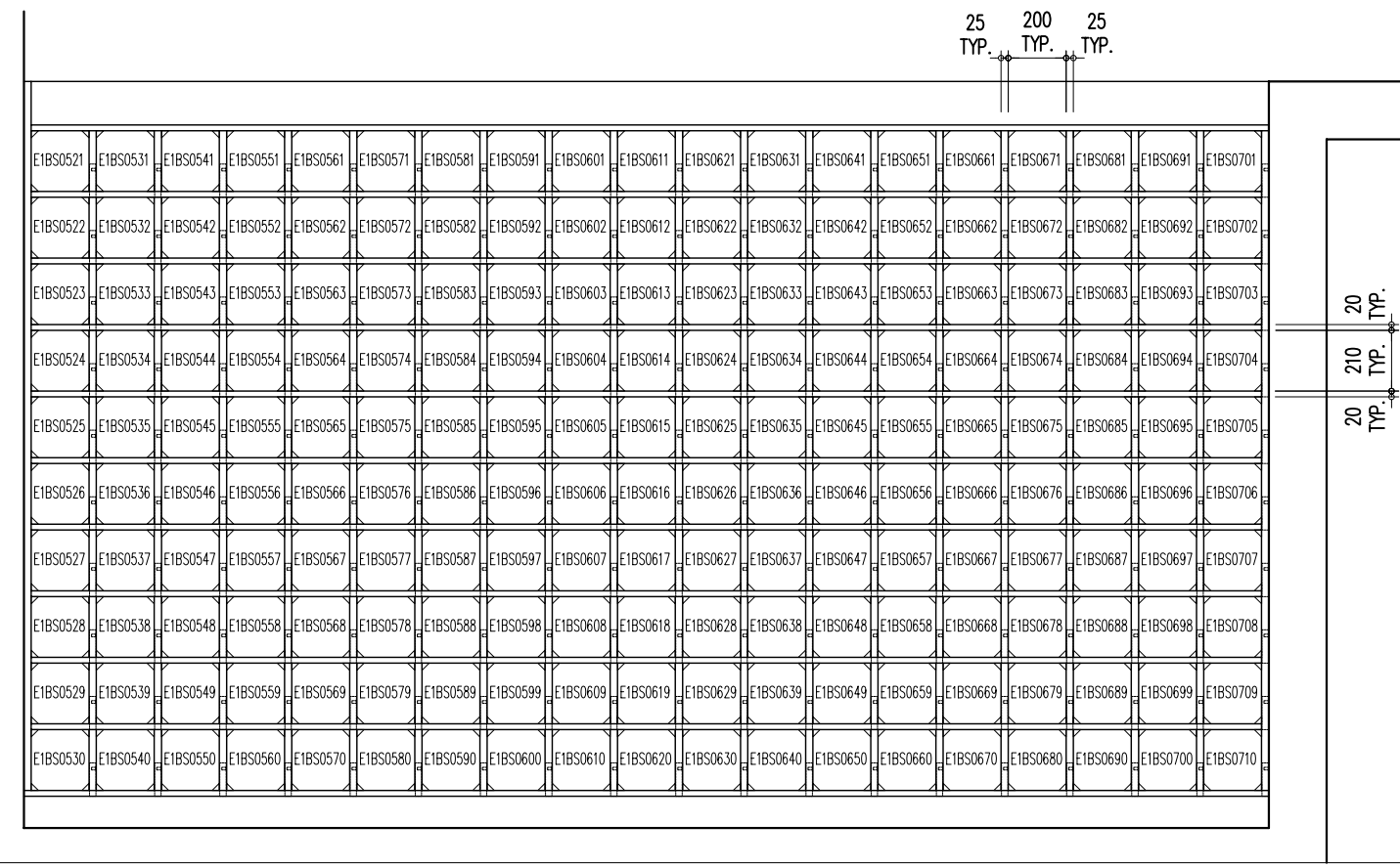
E1BS0521 ~ E1BS0710 一樓立面圖 A
