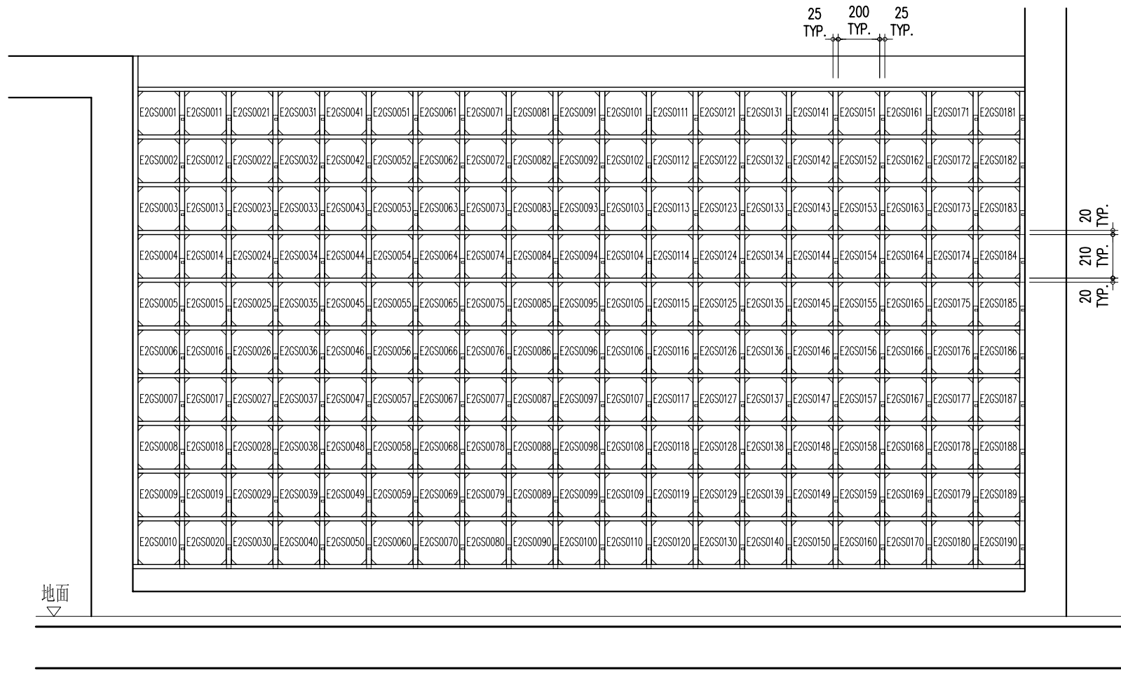
E2GS0001~E2GS0190 二樓立面圖 A
