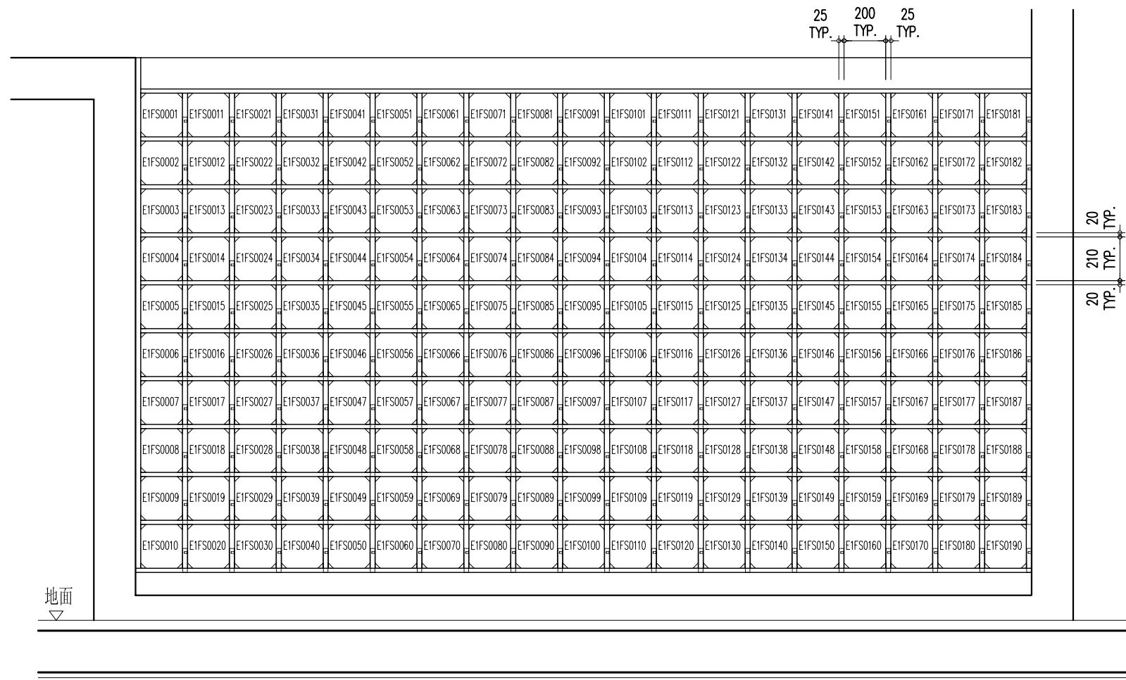
E1FS0001 ~ E1FS0190 一樓立面圖 A
