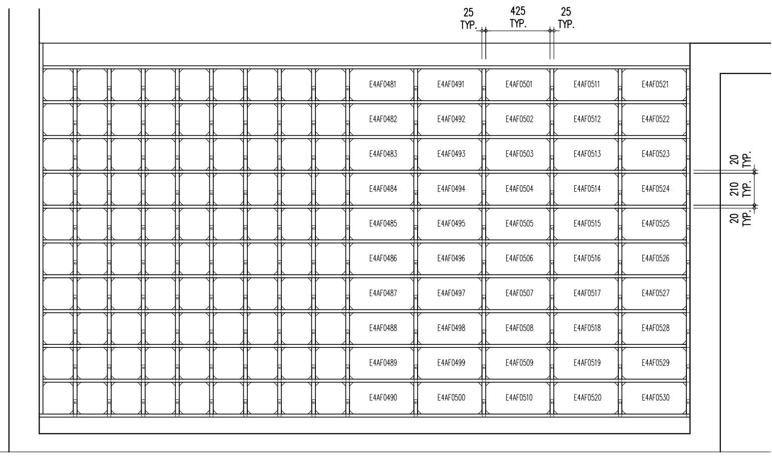
E4AF0481 ~ E4AF0530 四樓立面圖 A
