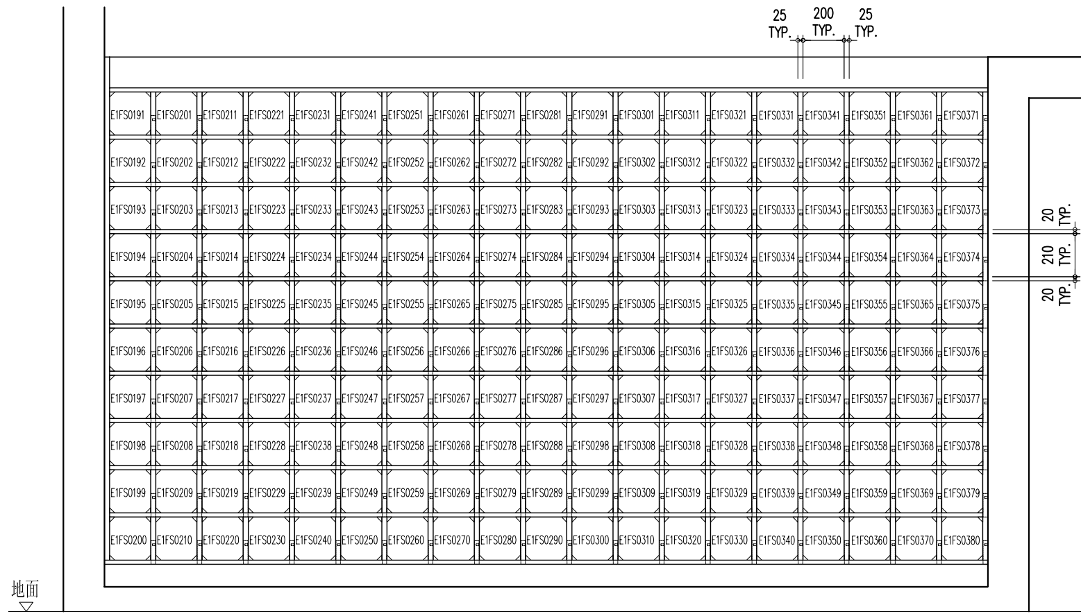
E1FS0191 ~ E1FS0380 一樓立面圖 A
