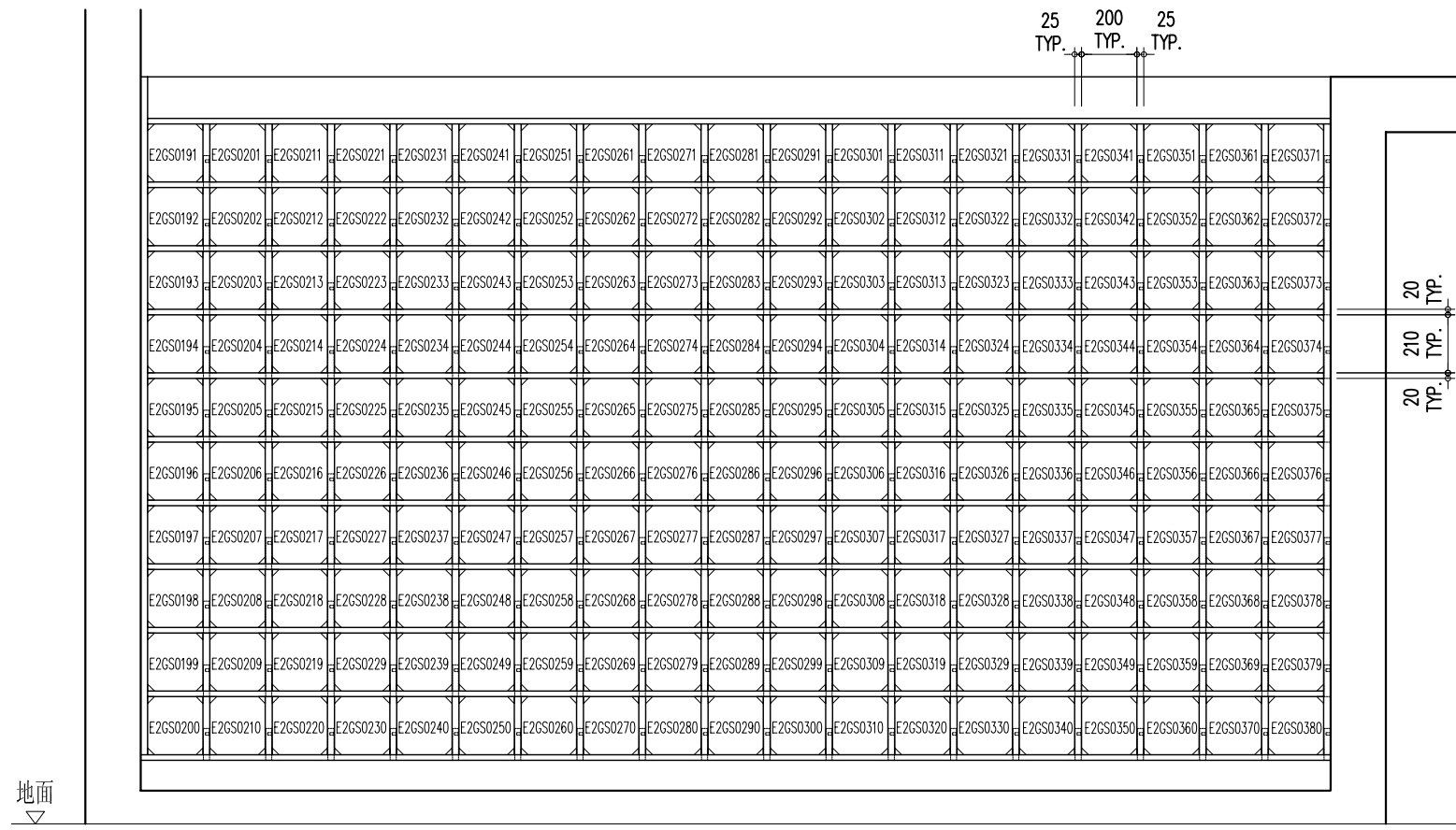
E2GS0191~ E2GS0380 二樓立面圖 A
