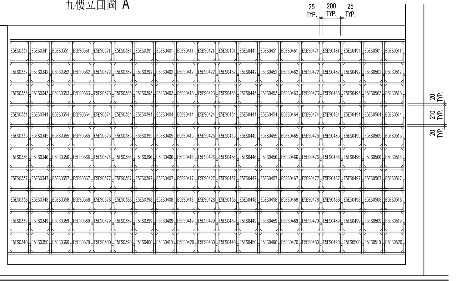
E5ES0331 ~ E5ES0520 五樓立面圖 B
