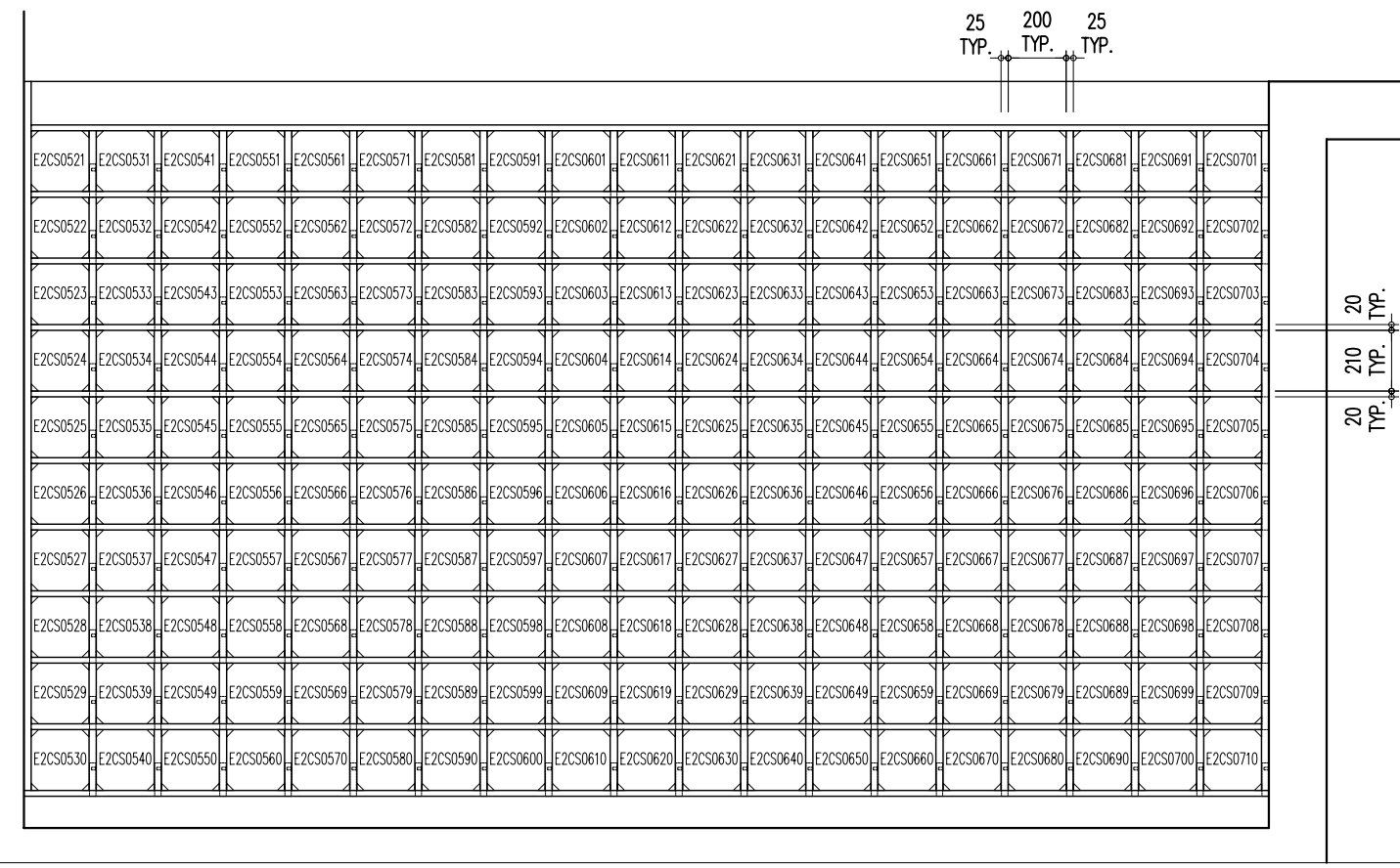
E2CS0521 ~ E2CS0710 二樓立面圖 A
