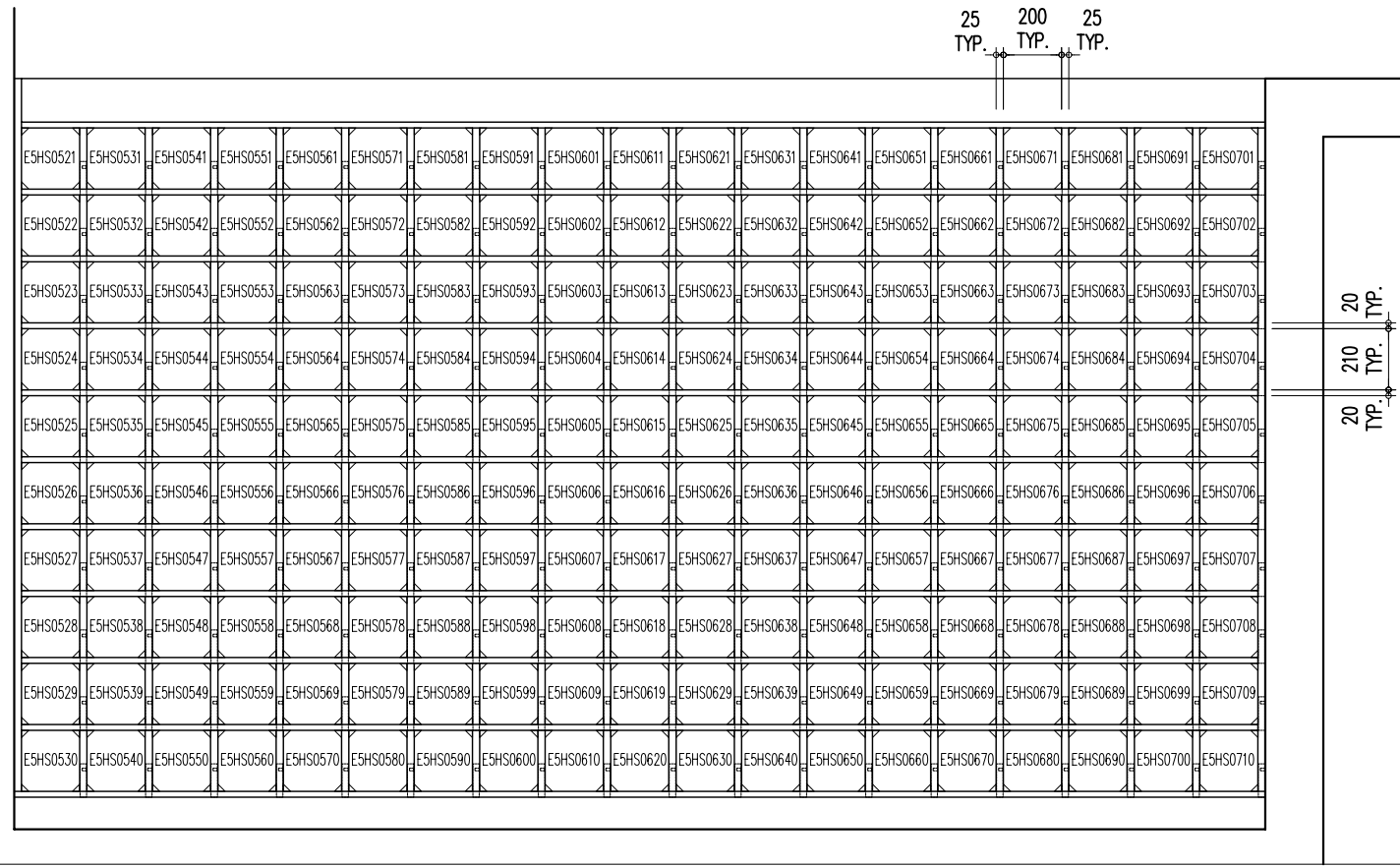
E5HS0521~E5HS0710 五樓立面圖 A
