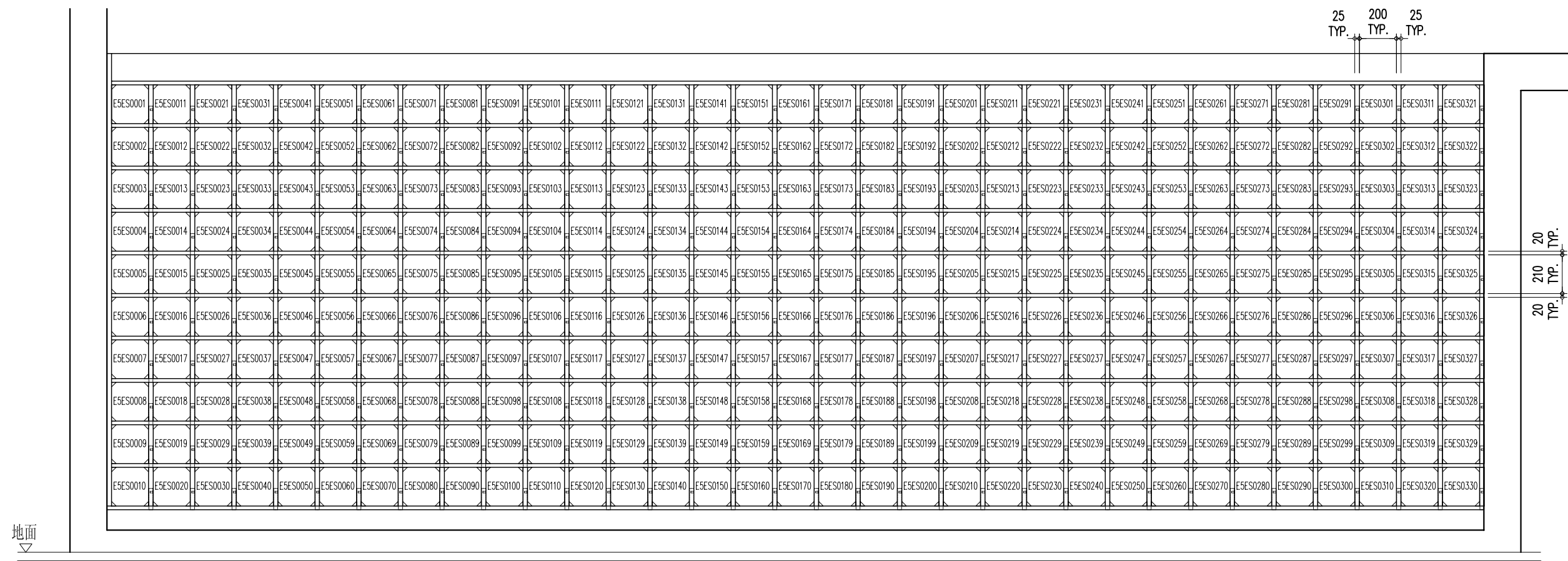
E5ES0001 ~ E5ES0330 五樓立面圖 A
