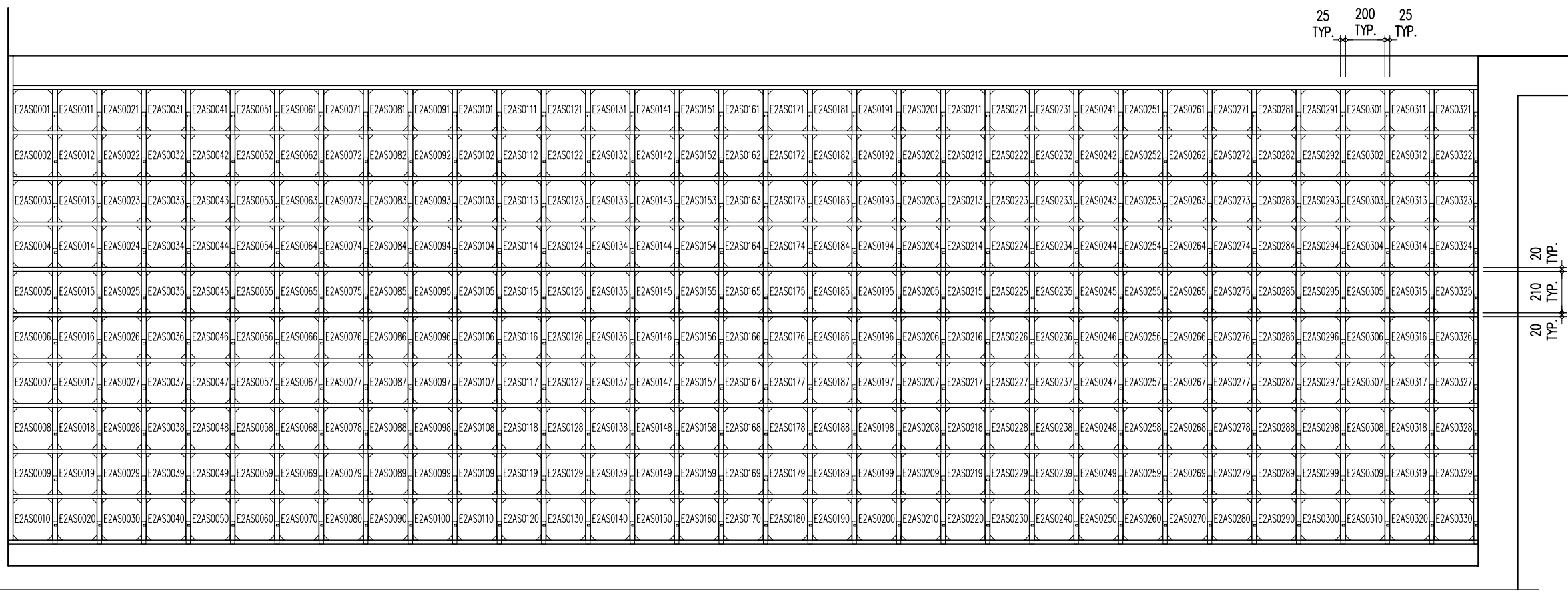
E2AS0001 ~ E2AS0330 二樓立面圖 A
