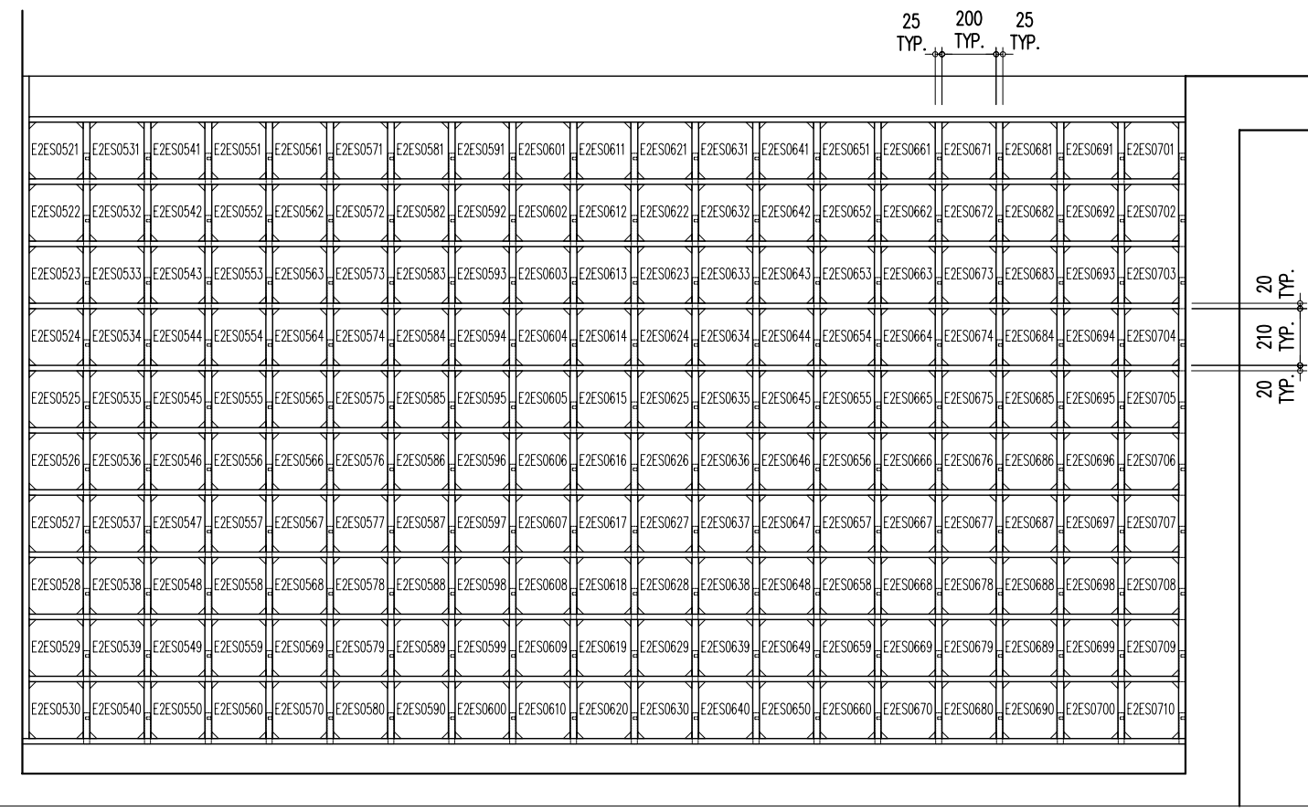
E2ES0521 ~ E2ES0710 二樓立面圖 A
