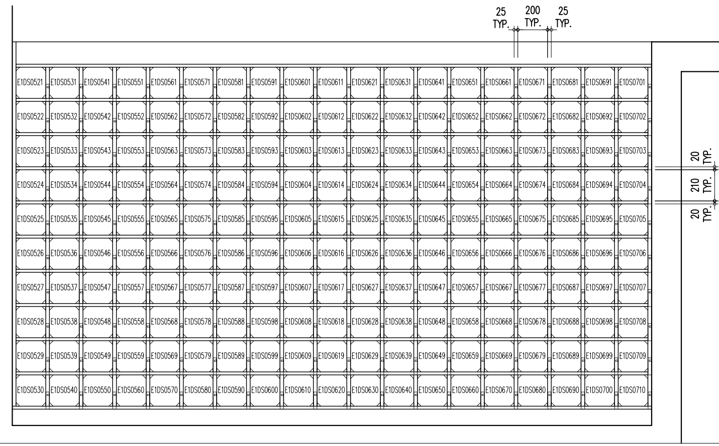
E1DS0521 ~ E1DS0710 一樓立面圖 A
