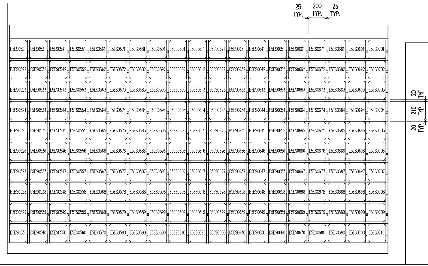
E5ES0521 ~ E5ES0710 五樓立面圖 A
